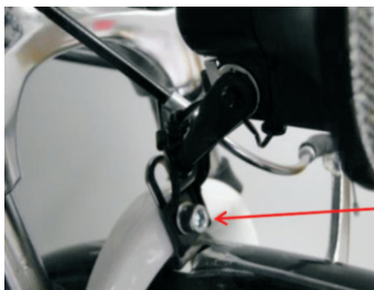
ŚRUBA MOCUJĄCA UCHWYT LAMPY I BŁOTNIKA PRZEDNIEGO
