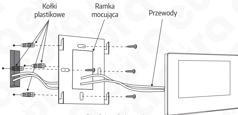
Rys. 2. Instalacja monitora
