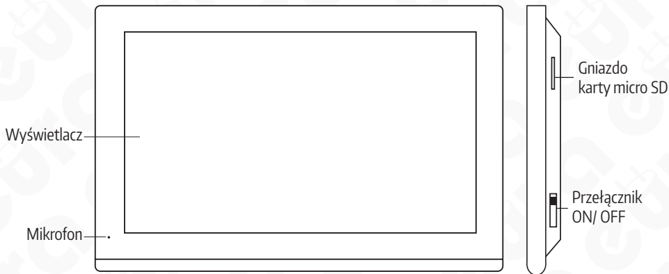
Rys. 1. Budowa monitora
