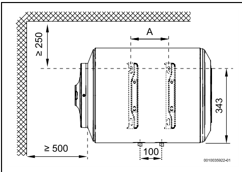
Rys. 3 Wymiary w mm (montaż ścienny, poziomy, TR1000...H)
