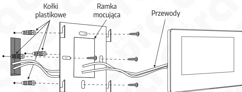
Rys. 2. Instalacja monitora
