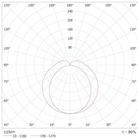
KANLUX S.A. (kat 36650) AKVO IP44 15W-NW-W S / Krzywa rozsyłu światła (biegunowo)
